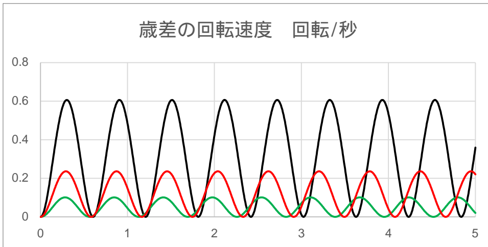
横軸 時間 秒 縦軸 歳差の回転速度 回転/秒
