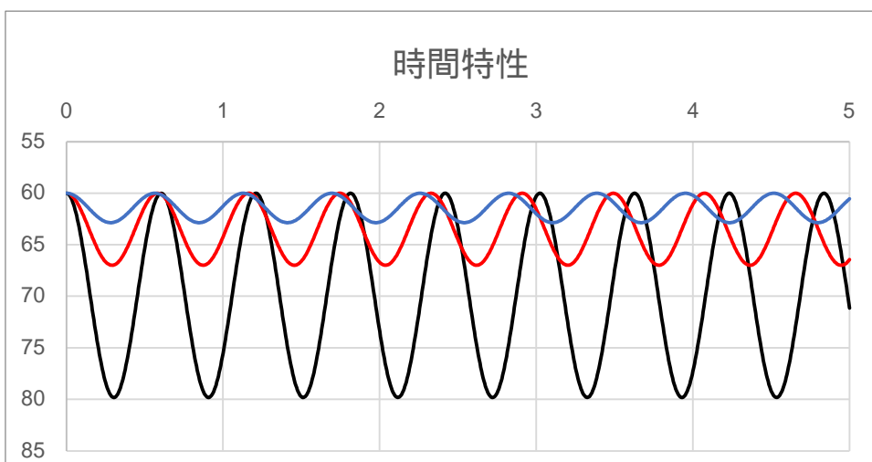
横軸 時間 秒 縦軸 章動の角度 度
